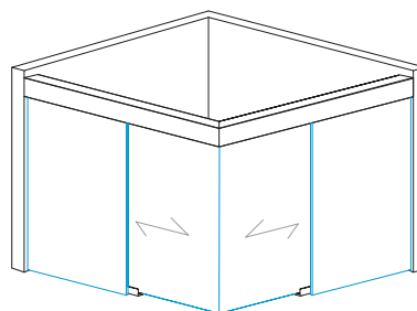
TR-R90-1000 Zostava rohová 90° Corner 90° set
